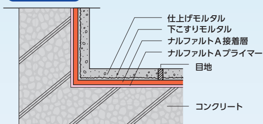
施工断面図
