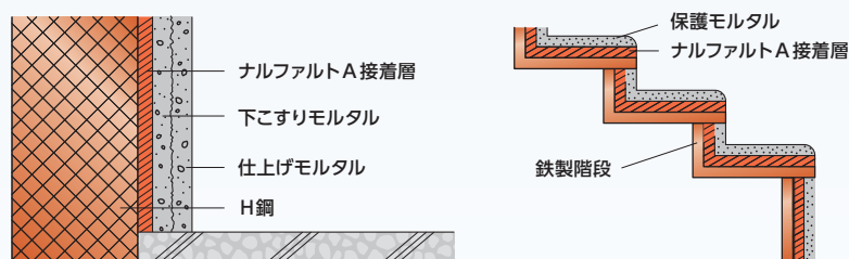
施工断面図
